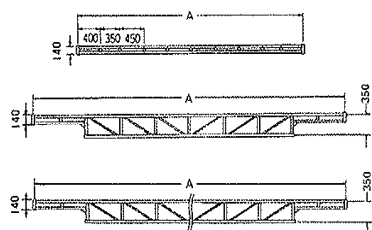
品名 梁棒
