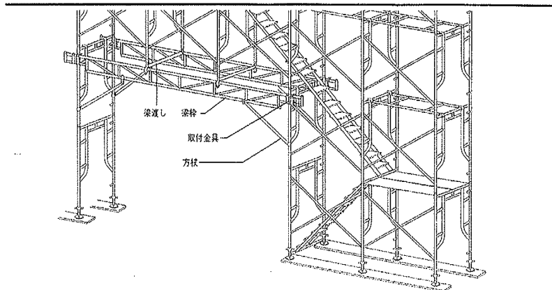
品名 梁棒
